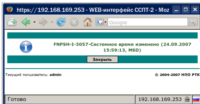
Рисунок 2.22: Вывод диагностического сообщения в WEB интерфейсе ССПТ-2
