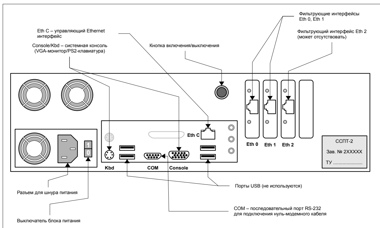
Рисунок 3.57: ССПТ-2 в корпусе 2U 19". Задняя панель
