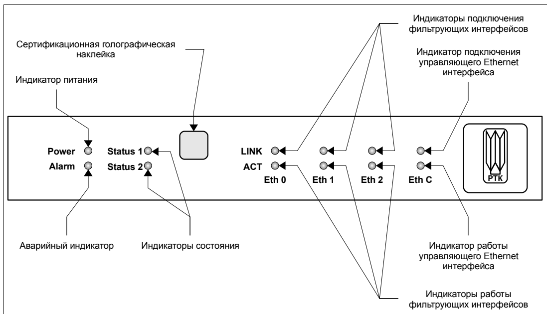
Рисунок 3.58: ССПТ-2 в настольном исполнении. Передняя панель
