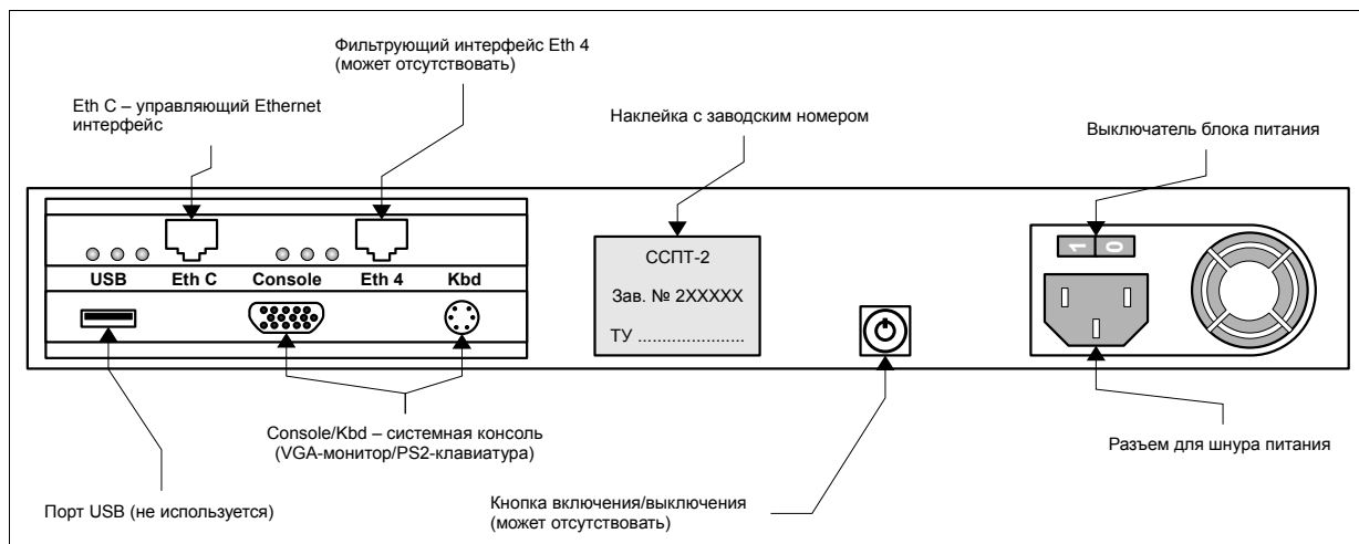
Рисунок 3.55: ССПТ-2 в корпусе 1U 19". Задняя панель
