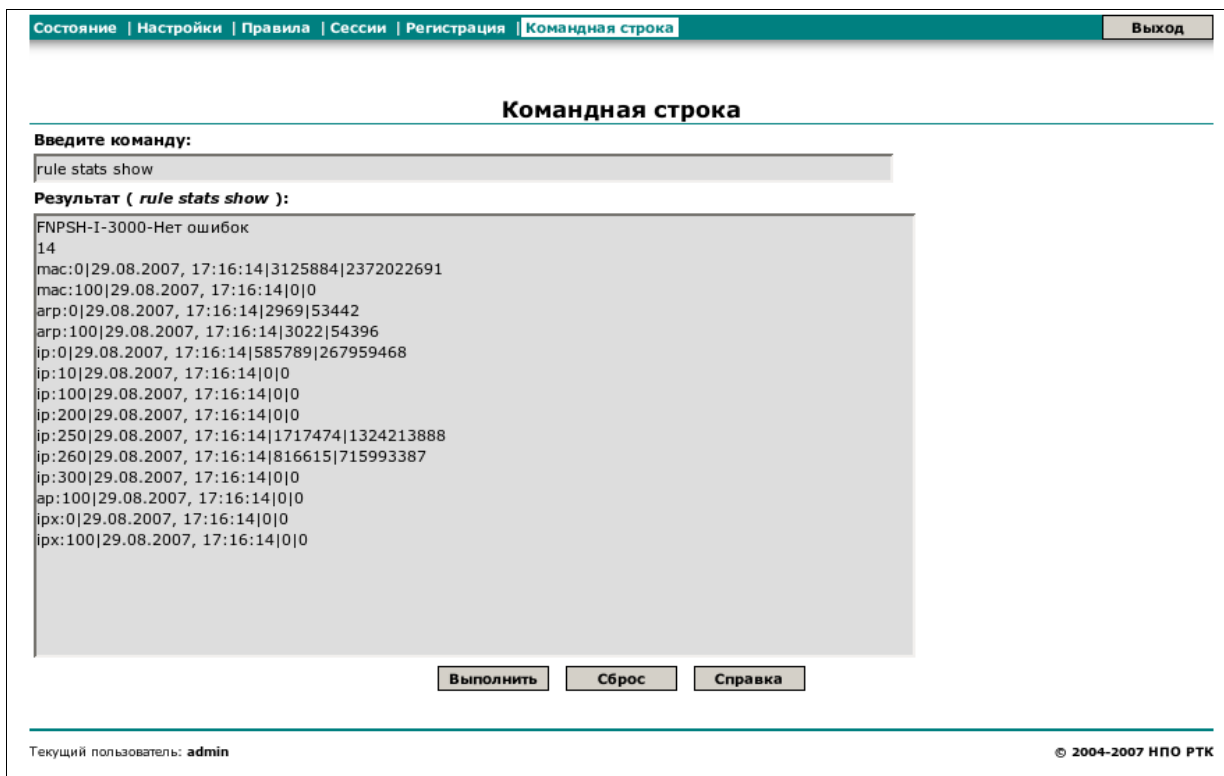
Рисунок 2.21: Раздел "Командная строка"
