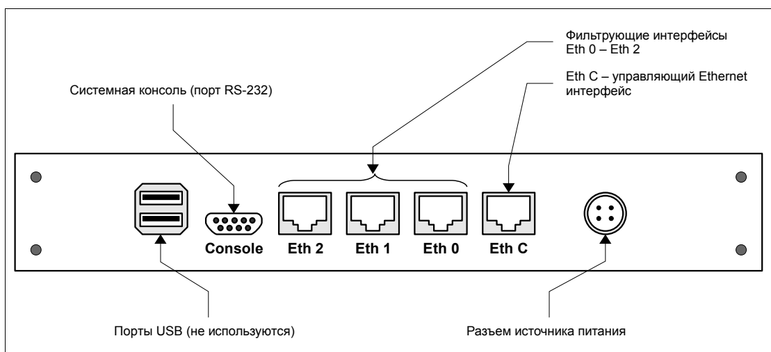
Рисунок 3.59: ССПТ-2 в настольном исполнении. Задняя панель
