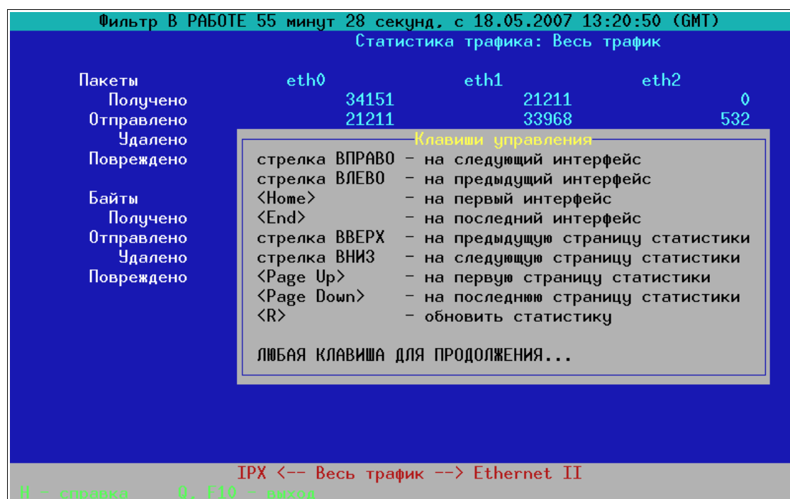
Рисунок 3.45: Состояние пакетного фильтра и статистика трафика
