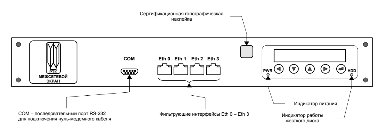
Рисунок 3.54: ССПТ-2 в корпусе 1U 19". Передняя панель
